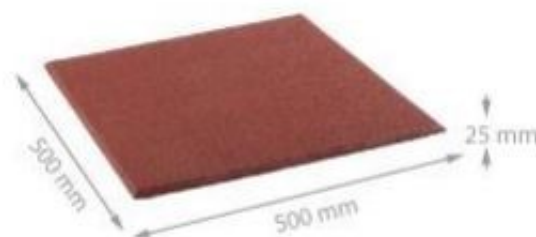
Rys. 1. Wymiary urządzenia
